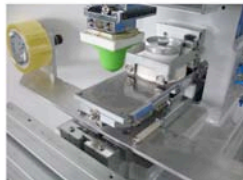
Klischeebeweger (Tamponreinigung darunter)
